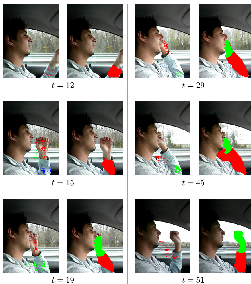
FIG. 8.10: Résultats de la méthode suivi sur la séquence d'un conducteur. Les observations sont les clusters en mouvement obtenus avec le détecteur de la partie I. À chaque instant, les observations sont montrées sur l'image de gauche et le masque des objets suivis est visible sur l'image de droite.
