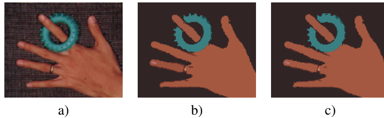
FIG. 4.8: Validation du clustering "pseudo balloon mean shift" sur l'image d'une main. a) Image originale ; b) Résultat de la segmentation avec l'algorithme "variable bandwidth mean shift" ; c) Résultat avec l'algorithme "pseudo balloon mean shift".
