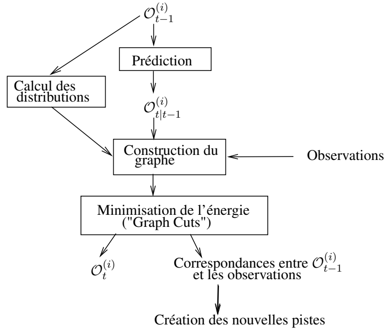
FIG. 8.2: Principe de l'algorithme de suivi.
