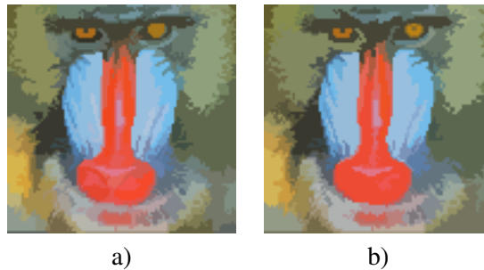
FIG. 4.11: Ordre de traitement des espaces de caractéristiques. Résultats sur l'image d'un singe du clustering "pseudo balloon mean shift" avec les bandes passantes obtenues en traitant les domaines dans les ordres suivants : a) abscisse, ordonnée, canal rouge, canal vert, canal bleu ; b) canal bleu, canal vert, canal rouge, ordonnée, abscisse.
