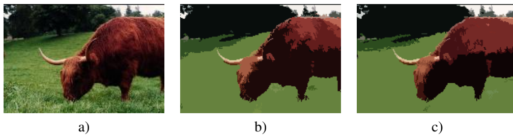
FIG. 4.9: Validation du clustering "pseudo balloon mean shift" sur l'image d'un taureau. a) Image originale ; b) Résultat de la segmentation avec l'algorithme "variable bandwidth mean shift" ; c) Résultat avec l'algorithme "pseudo balloon mean shift".
