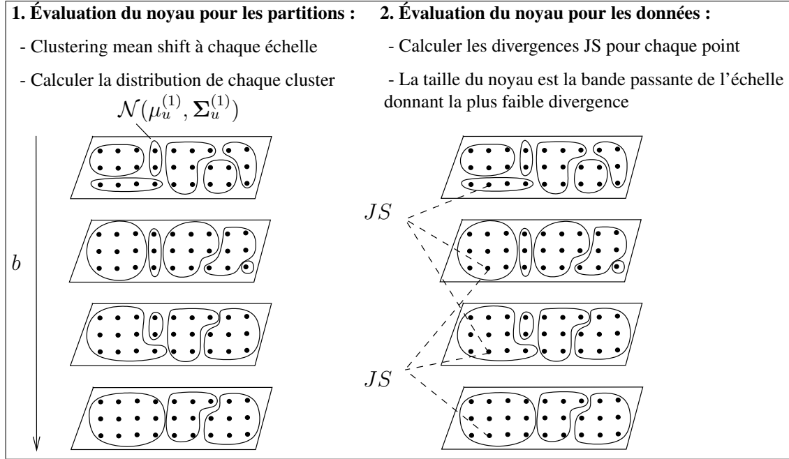
FIG. 4.1: Schéma représentant une itération de notre algorithme.
