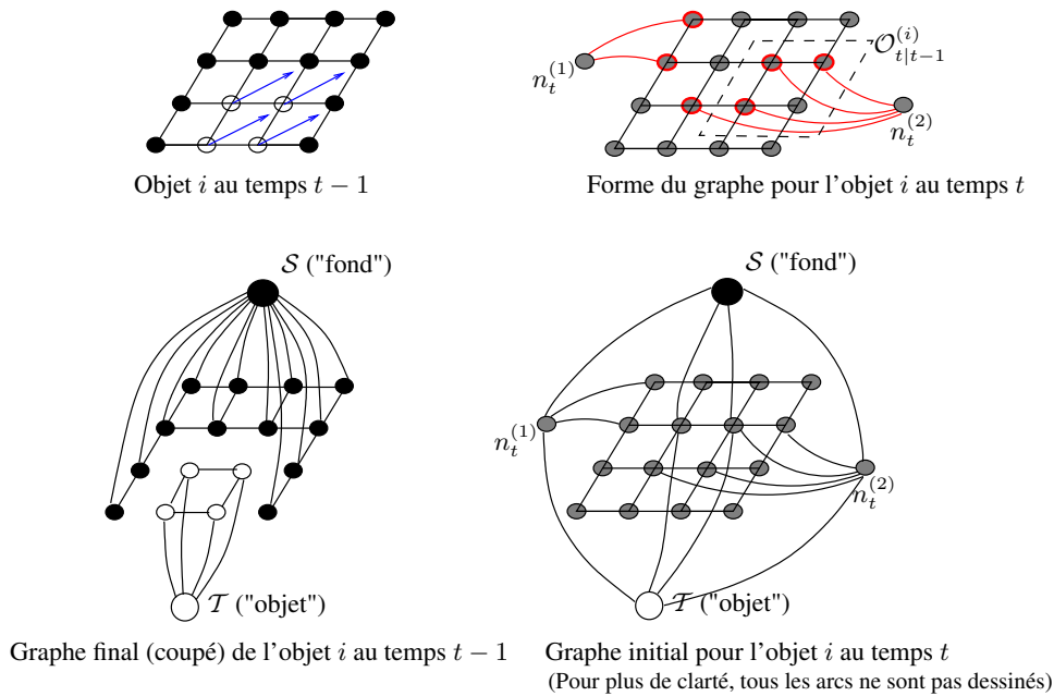
FIG. 8.3: Présentation du graphe utilisé. (a) Résultat de la minimisation d'énergie à l'instant t - 1 . Seuls les sommets correspondant aux pixels de l'image sont montrés. L'étiquette des nœuds blancs est "objet" et celle des nœuds noirs est "fond". En bleu est montré en chaque pixel de l'objet le vecteur de mouvement moyen qui permet la prédiction. (b) Graphe coupé correspondant à (a) avec les terminaux. Les arcs coupés ne sont pas dessinés. (c) Forme du graphe à l'instant t . Les terminaux et leurs arcs associés ne sont pas montrés. Les nœuds (n_t^{(1)}) et (n_t^{(2)}) associés aux deux observations détectées \mathcal{M}_t^{(1)} et \mathcal{M}_t^{(2)} sont ajoutés à l'ensemble des sommets correspondant aux pixels. Les sommets en rouge représentent les pixels appartenant aux observations. Les arcs reliant ces sommets aux sommets correspondant aux observations apparaissent en rouge. Cette figure montre également les sommets appartenant à la prédiction. (d) Graphe avec les terminaux associés à (c). Pour des raisons de lisibilité, tous les arcs entre les terminaux et les autres sommets ne sont pas montrés.
