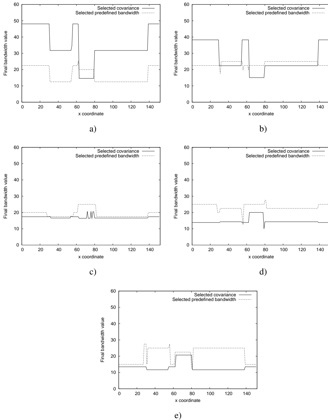
FIG. B.3: Valeurs finales des bandes passantes pour tous les points situés sur la ligne au milieu de l'image d'une main a) domaine correspondant aux abscisses b) domaine correspondant aux ordonnées c) canal rouge d) canal vert and e) canal bleu.
