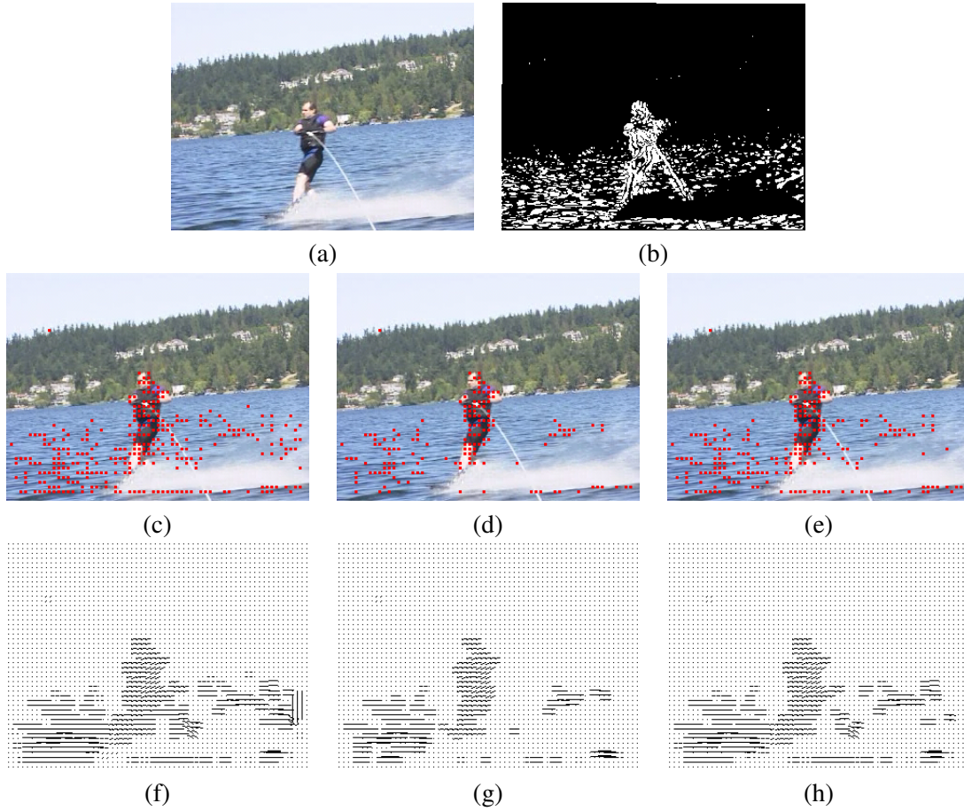
FIG. 2.4: Construction de la grille de points (deuxième ligne) et calcul du flot optique (troisième ligne) sur l'image 108 de la séquence de ski nautique. (a) Image initiale. (b) Carte des pixels en mouvement. (c) Grille restreinte uniquement aux pixels en mouvement (les vecteurs de mouvement sont montrés sur l'image (f)). (d) Grille finale obtenue après validation des vecteurs de mouvement par un test de corrélation (seuil = 0.5). (les vecteurs de mouvement sont montrés sur l'image (g)). (e) Grille finale obtenue après validation des vecteurs de mouvement par un test statistique (les vecteurs de mouvement sont montrés sur l'image (h)).
