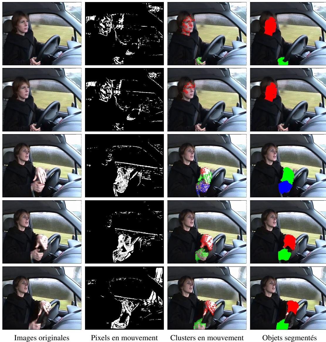
FIG. 5.3: Résultats de la détection sur la séquence d'une conductrice pour les images 16, 17, 40, 42 et 47
