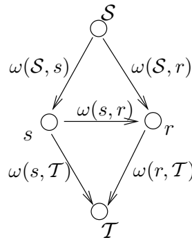
FIG. 6.5: Capacité des arcs reliant les sommets mutuellement voisins.
