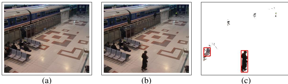
FIG. 8.5: Observations obtenues par soustraction de fond. (a) Image de référence. (b) Image courante. (c) Résultat de la soustraction de fond (les pixels en noir sont les pixels ayant changé) et observations déduites (régions entourées d'une boîte englobante rouge).
