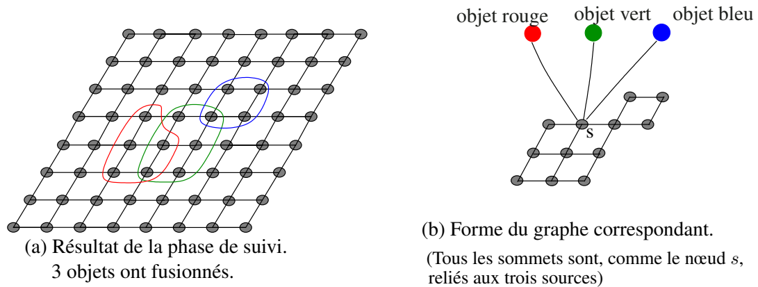
FIG. 8.4: Présentation du graphe utilisé. (a) Résultat de l'algorithme de suivi. Trois objets se superposent. (b) Forme du graphe correspondant à la deuxième fonction d'énergie. Il contient 3 terminaux (3 sources), chacun relié à l'ensemble des pixels. Pour plus de clarté, tous les arcs ne sont pas montrés.
