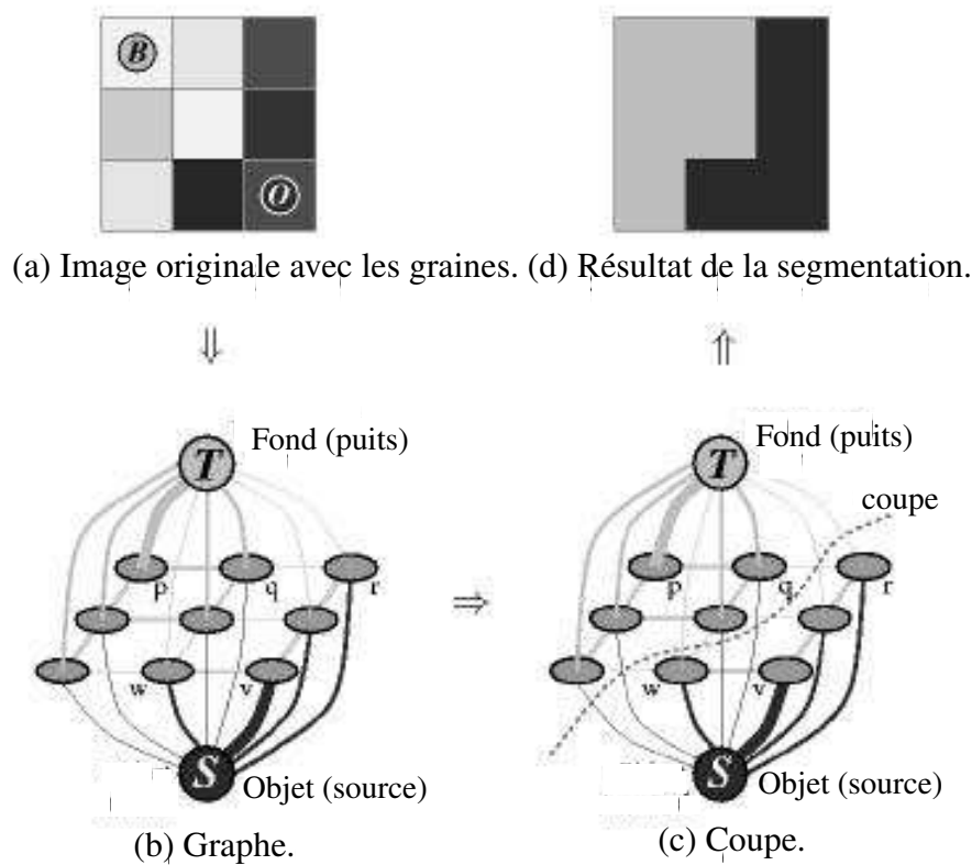
FIG. 6.7: Exemple de graphe et de segmentation. La capacité de chaque arc est traduite par son épaisseur. Cette figure provient de [Boykov 01a].
