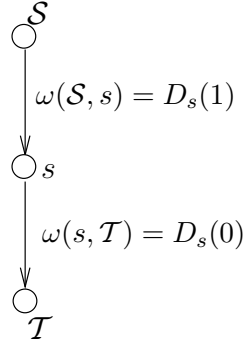
FIG. 6.4: Capacité des arcs reliant les terminaux aux nœuds du graphe.
