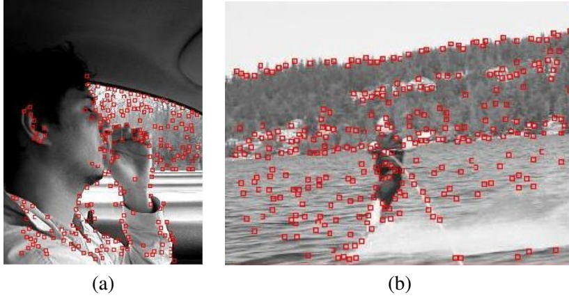
FIG. 2.3: Résultat du détecteur de coin Harris sur a) l'image 16 de la séquence de conducteur b) l'image 108 de la séquence ski nautique.
