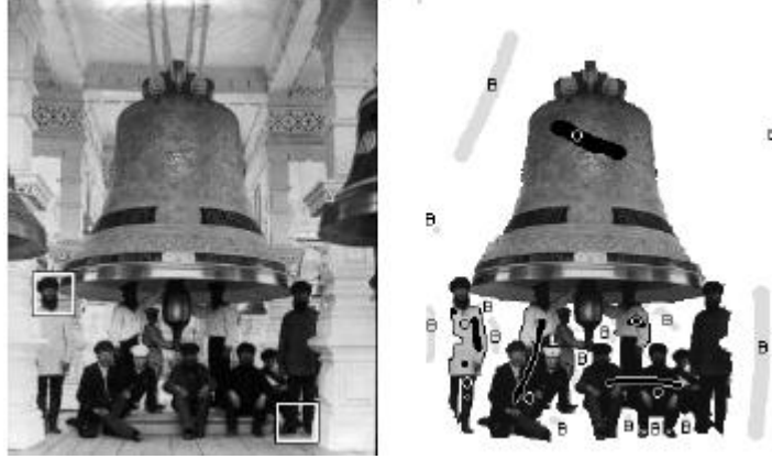
FIG. 6.6: Graines placées à l'extérieur ("B") et à l'intérieur de l'objet ("O") à segmenter : à gauche, l'image originale, à droite, le résultat de la segmentation et les graines. Cette figure provient de [Boykov 01a].
