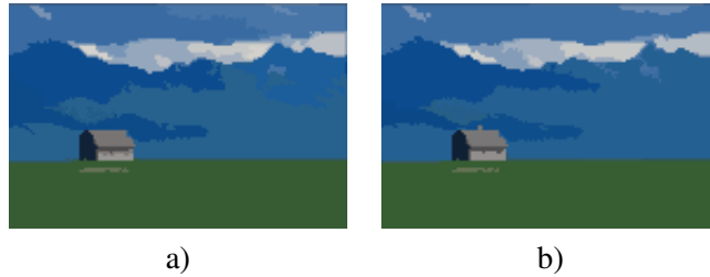
FIG. 4.10: Ordre de traitement des espaces de caractéristiques. Résultats sur l'image d'un chalet du clustering "pseudo balloon mean shift" avec les bandes passantes obtenues en traitant les domaines dans les ordres suivants : a) abscisse, ordonnée, canal rouge, canal vert, canal bleu ; b) canal bleu, canal vert, canal rouge, ordonnée, abscisse.
