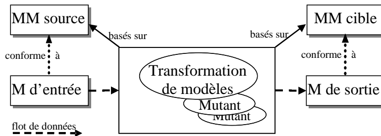
Figure 3-2 – Processus de transformation de modèles avec une transformation et ses mutants
