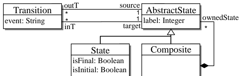
Figure 2-3 - Méta-modèle de machines à états composites
