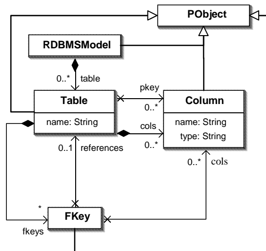
Figure 4-5 - Version relâchée du méta-modèle RDBMS
