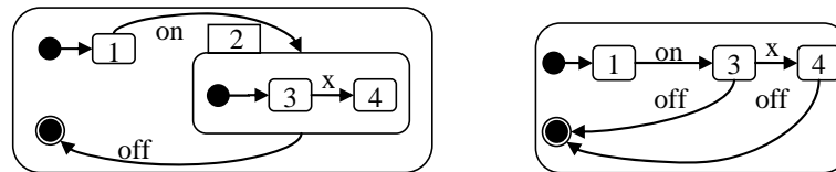
Figure 2-5 - Exemples de modèles de machines à états
