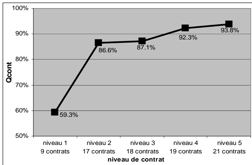
Figure 5-17 – Progression du score de mutation pendant l'amélioration des contrats.
