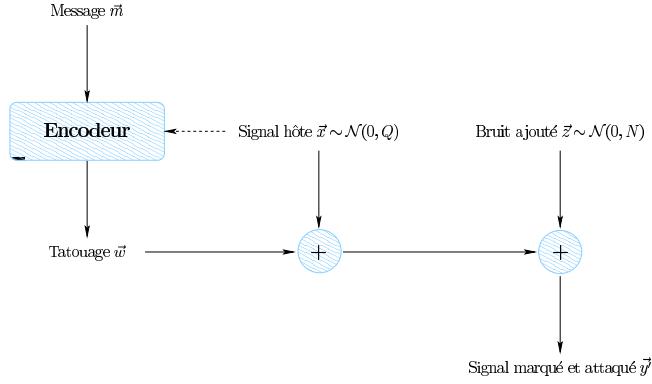
FIG. 1: Le tatouage vu comme de la communication avec information adjacente
