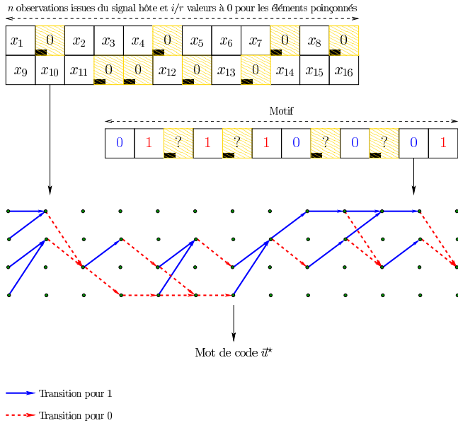
(b) Décodage du signal hôte grâce à un algorithme de Viterbi avec un treillis dont seuls les transitions compatibles avec le motif ont été conservées
