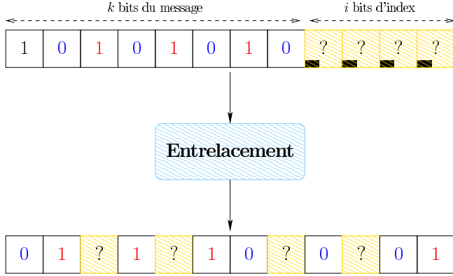
(a) Construction d'un motif pour le décodage de \vec{x}
