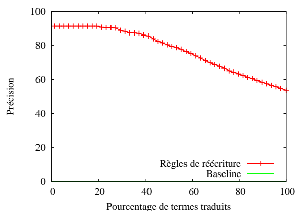
FIG. 7 – Performances de traduction du russe vers l'anglais
