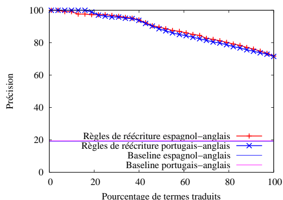
FIG. 5 – Performances de traduction portugais/espagnol vers anglais
