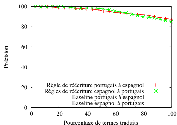
FIG. 4 – Performances de traduction espagnol - portugais
