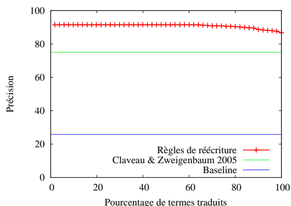
FIG. 3 – Performances de traduction de l'anglais vers français
