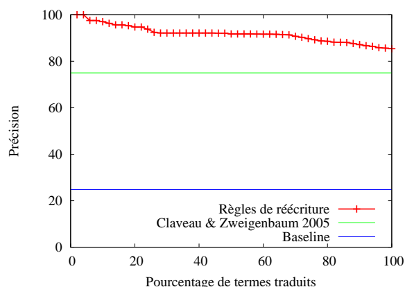
FIG. 2 – Performances de traduction du français vers l'anglais
