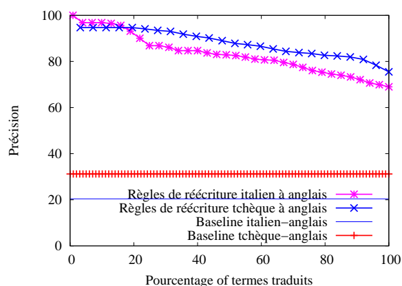
FIG. 6 – Performances de traduction de l'italien/tchèque vers l'anglais
