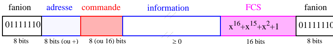
format général d'une trame HDLC
