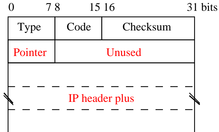
ICMP parameter error message
