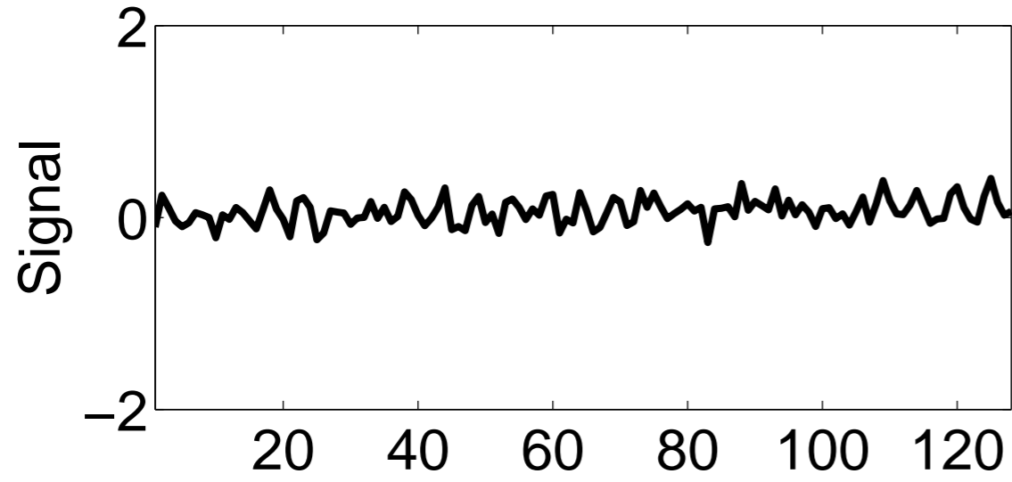
Signal genere par la base de cosinus
