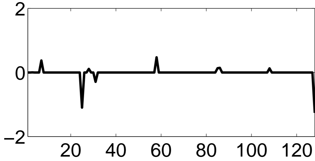
Coefficients sur la base de cosinus
