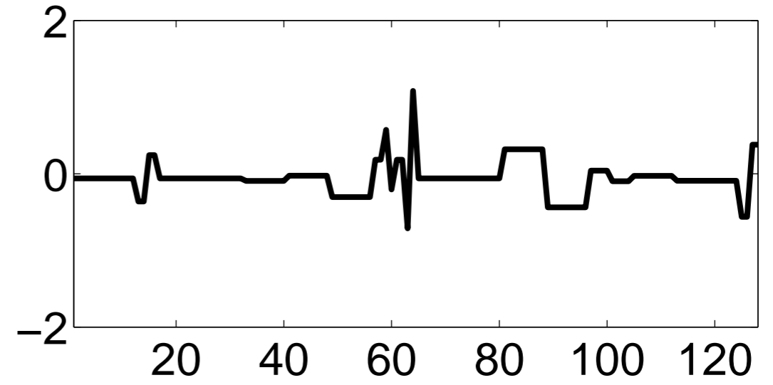
Signal genere par la base de Haar
