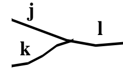
OR-join
