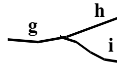
OR-fork
