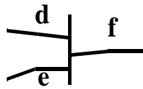
AND-join
