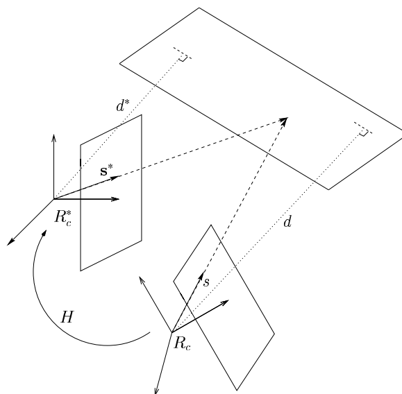
FIG. 1.8 – Principe de l'asservissement visuel 2D 1/2
